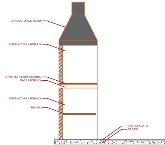
CORTE A'-A'
